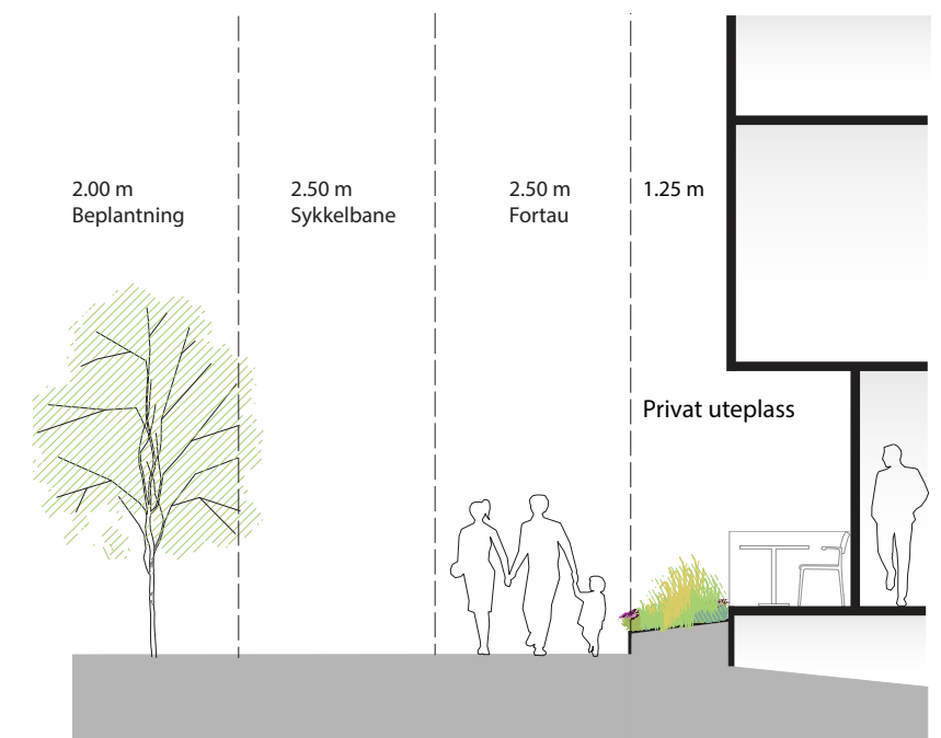
D. Prinsippsnitt som viser hvordan overganger mellom private og offentlige arealer kan tas opp med et plantefelt for å etablere en fin og tydelig overgang.
