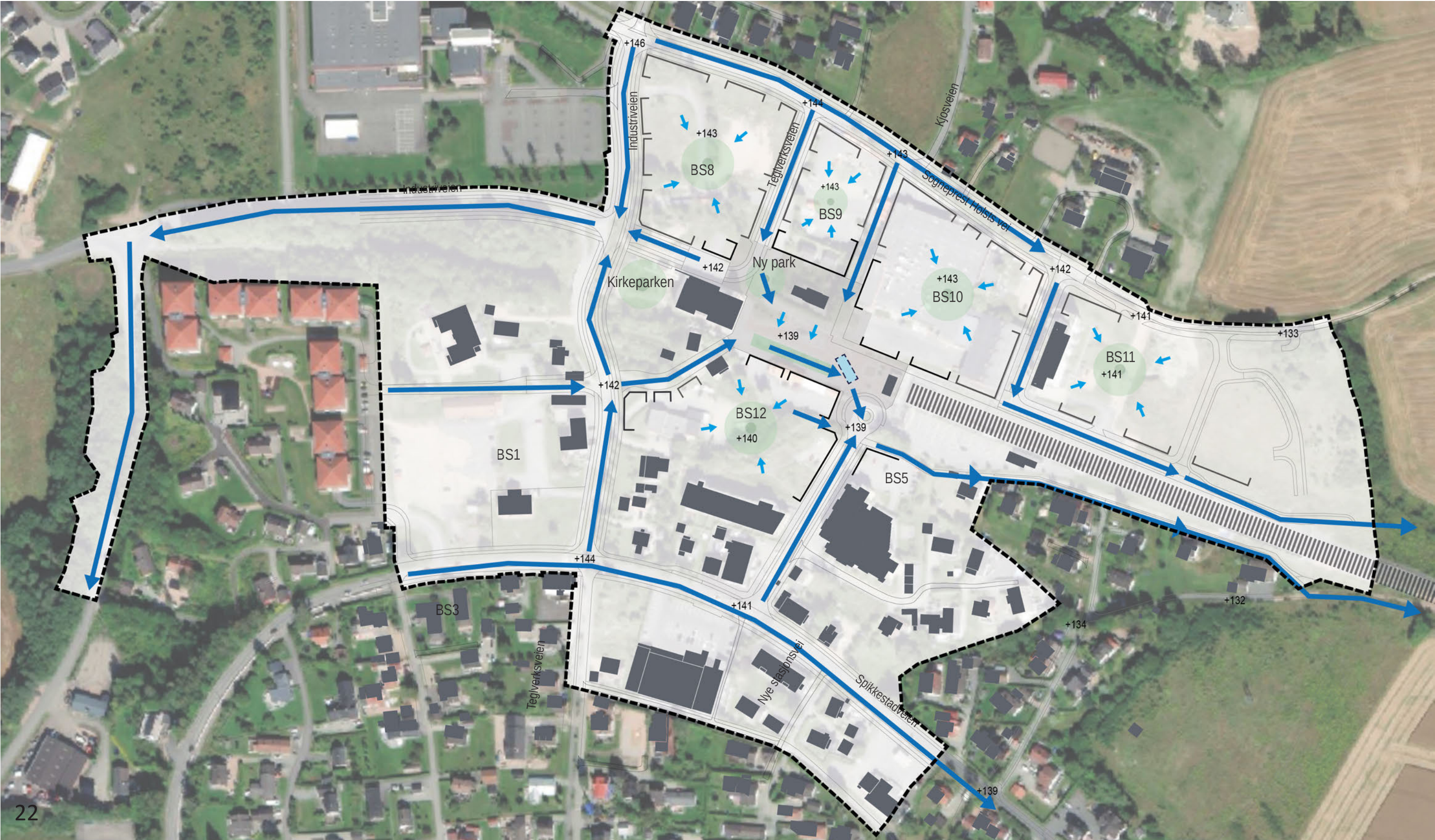
Illustrasjonen viser at overvannet håndteres i hvert kvartal og flomveier mot øst og mot kulturlandskapet.
