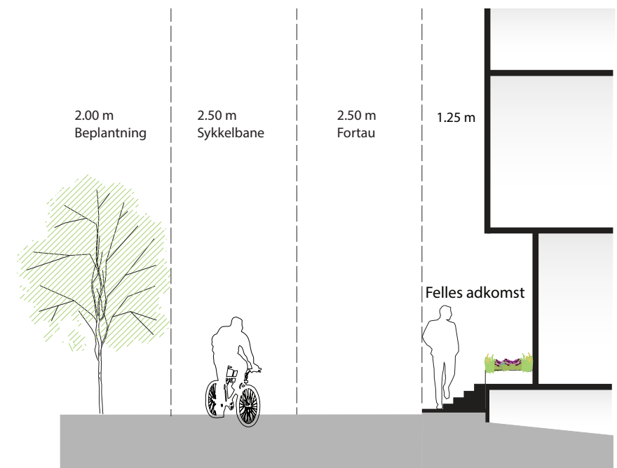
B. Prinsippsnitt som viser hvordan adkomstene kan markeres med en trapp og inntrukket inngangsparti.
