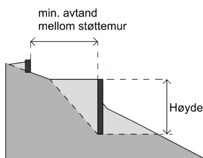
Figur 1b. Høyde på støttemur med fyllinger
