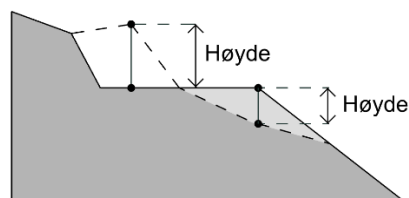
Figur 1c. Høyde på skjæring og fylling måles fra høyeste punkt og laveste punkt loddrett
